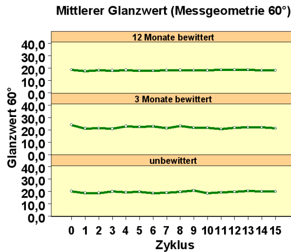
Abbildung 3 : Glanzwertänderungen im Stresstest (Messgeometrie 60°)
