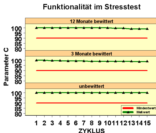
Abbildung 1 : Funktionalität im Stresstest
