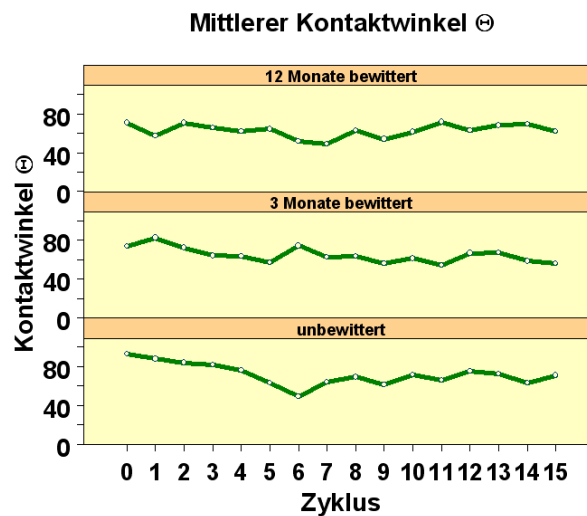
Abbildung 4 : Mittlerer Kontaktwinkel \Theta im Stresstest (Monitorfeld)
